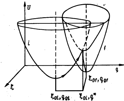
Рис. 16. Расположение поверхностей потенциальной энергии при квазибезбарьерном переходе
