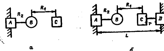
Рис. 26. Схема реакции присоединения в модели линейного комплекса:
