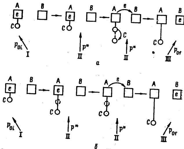
Рис. 19. Схема реакции электронного переноса, сопровождающейся изменением состояния внутримолекулярной степени свободы (состояния частицы C): а — случай квантовой внутримолекулярной степени свободы; б — случай классической внутримолекулярной степени свободы
