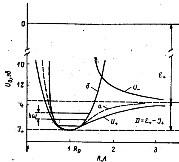
Рис. 4. Электронные термы иона \text{H}_2^+ :
